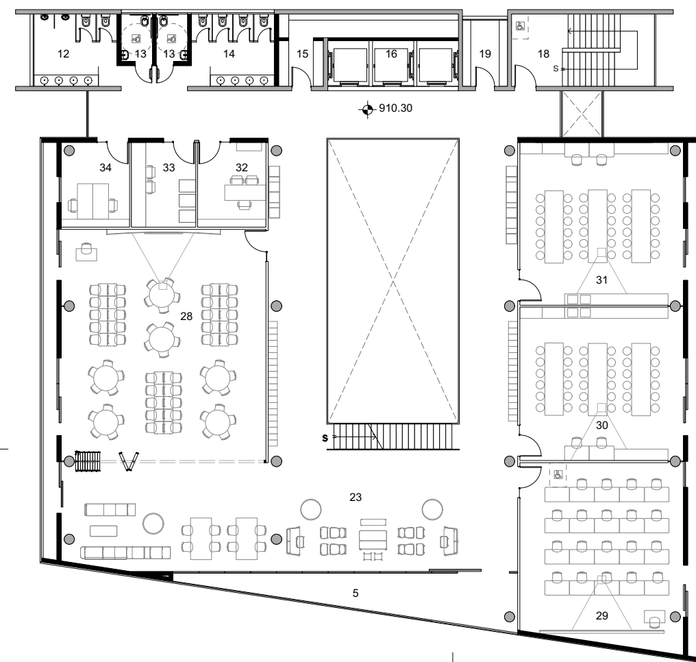
PLANTA DO QUARTO PAVIMENTO N 910.30 | ÁREA: 748.50m² | ESC 1:250
