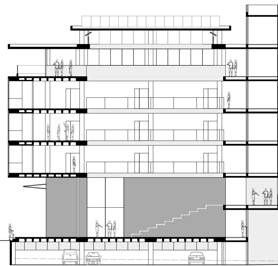
CORTE AA ESC 1:250
