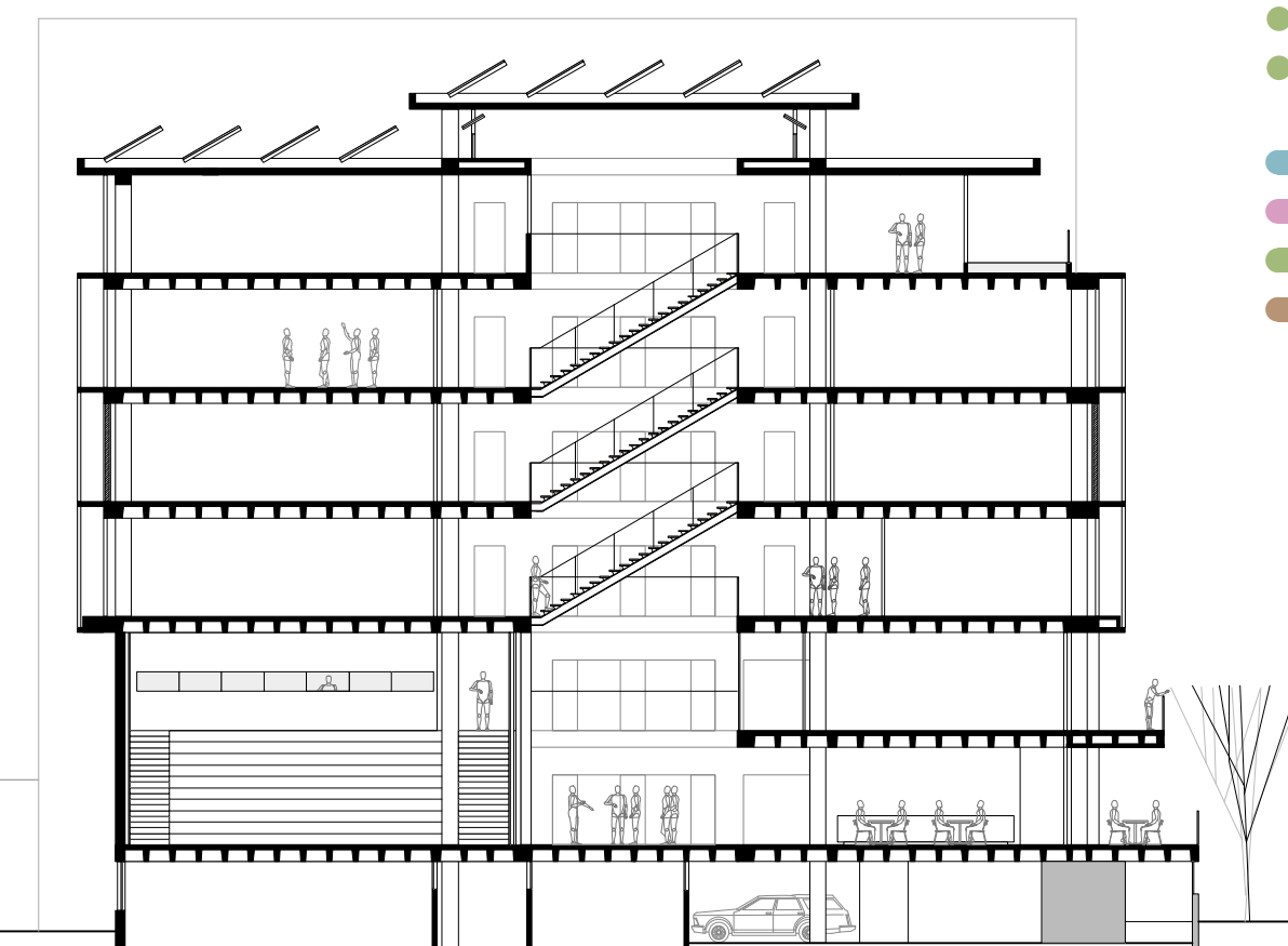
CORTE BB ESC 1:250
