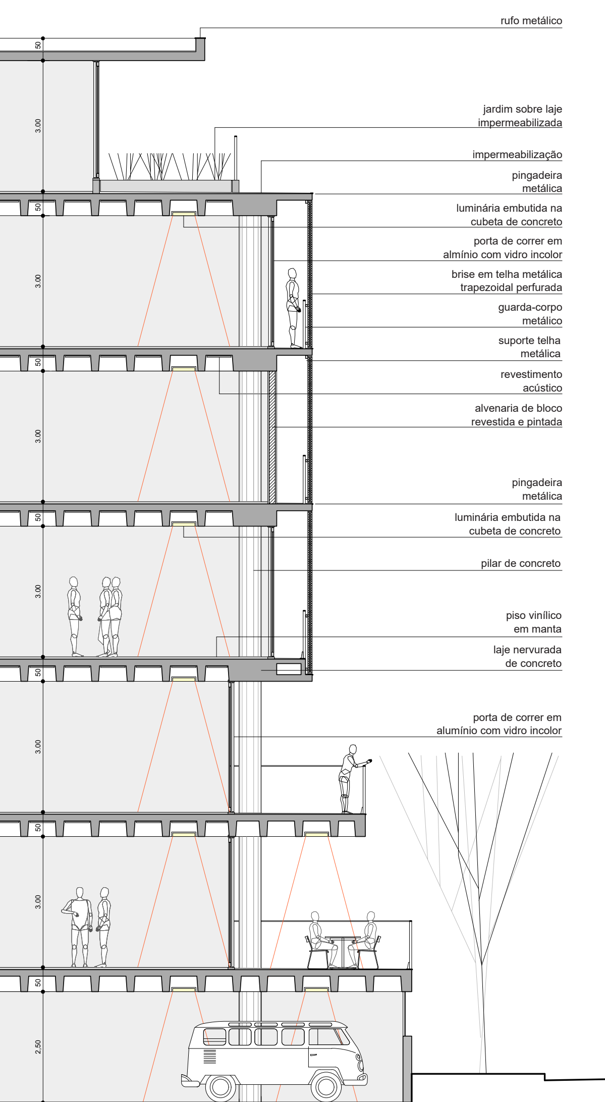
SEÇÃO AMPLIADA SEM ESCALA
