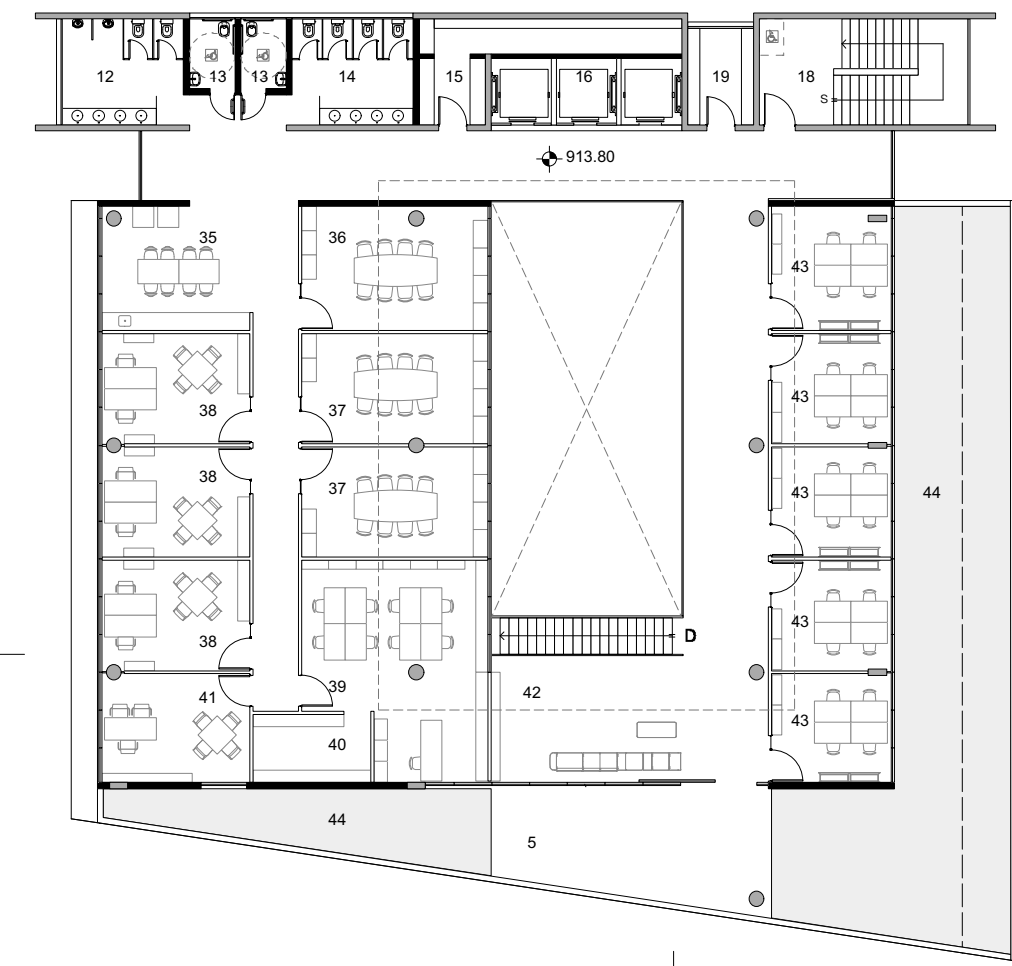
PLANTA DO QUINTO PAVIMENTO N 913.80 | ÁREA: 605.48m² | ESC 1:250
